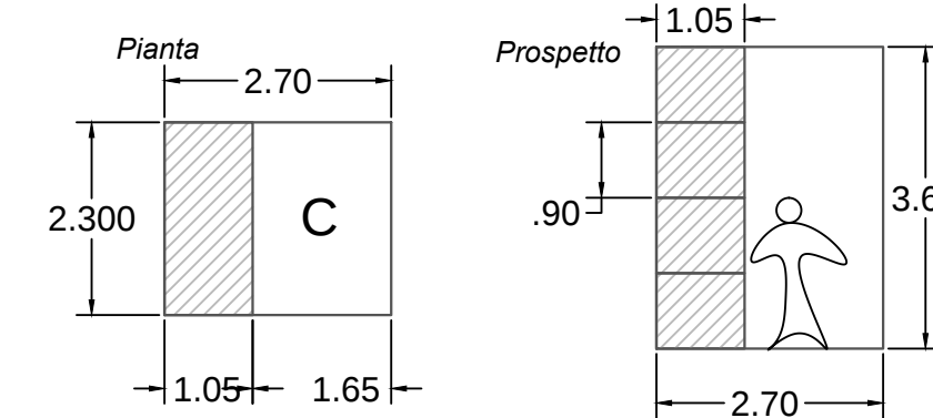
MODULO DI PROGETTO D 4 posti a terra - tomba ipogea
