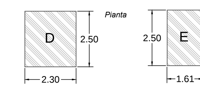
MODULO DI PROGETTO E 2 posti a terra - tomba ipogea
