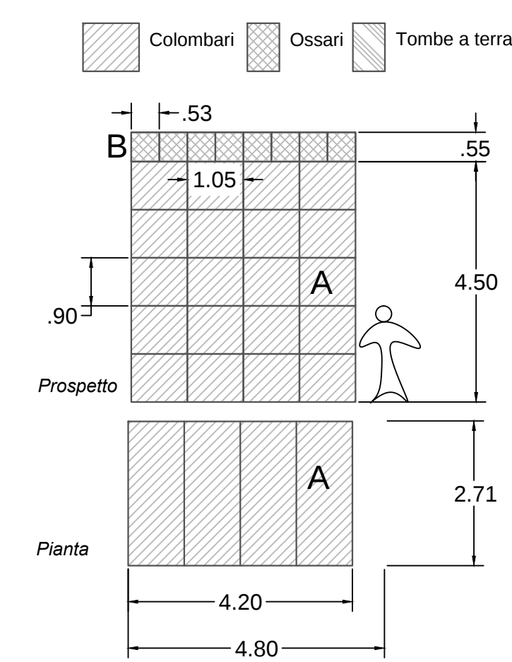
MODULO DI PROGETTO C 8 Colombari - Tomba di Famiglia
